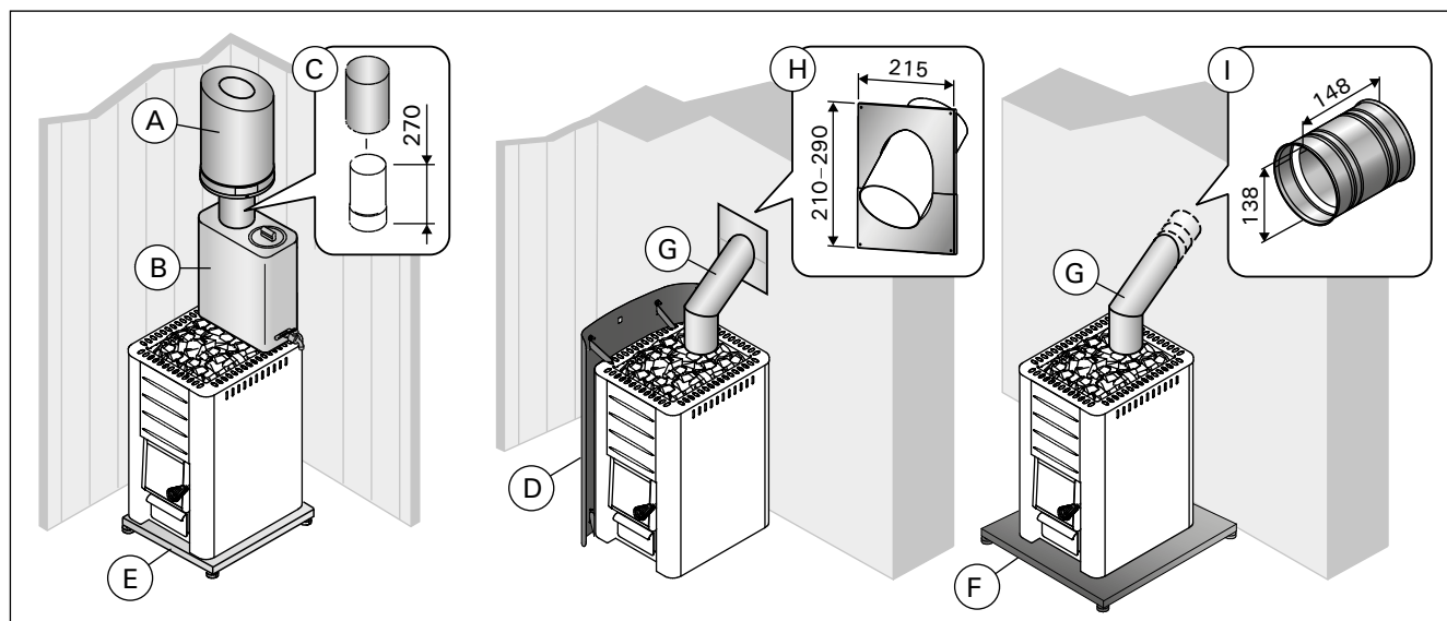
Figure 13. Accessoires (toutes les dimensions sont fournies en millimètres) Figura 13. Accessori (tutte le dimensioni sono espresse in millimetri)
