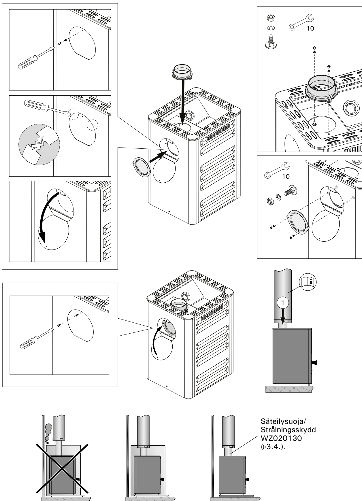
Kuva 11. Kiukaan liittäminen Harvia-teräspiippuun Bild 11. Anslutning av ugnen till Harvia stålkorsten
