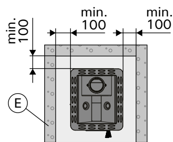
Obrázek 7. Bezpečné vzdálenosti pro topné těleso (všechny rozměry jsou uvedené v milimetrech) Figuur 7. Veiligheidsafstanden (alle afmetingen in millimeters)
