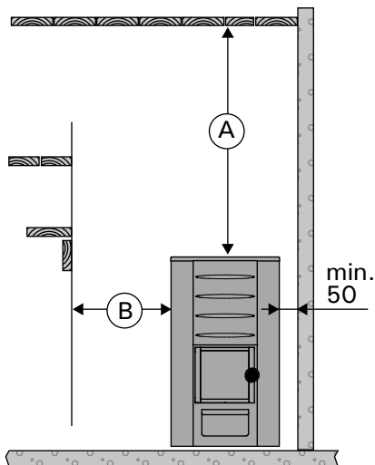
Obrázek 7. Bezpečné vzdálenosti pro topné těleso (všechny rozměry jsou uvedené v milimetrech) Figuur 7. Veiligheidsafstanden (alle afmetingen in millimeters)
