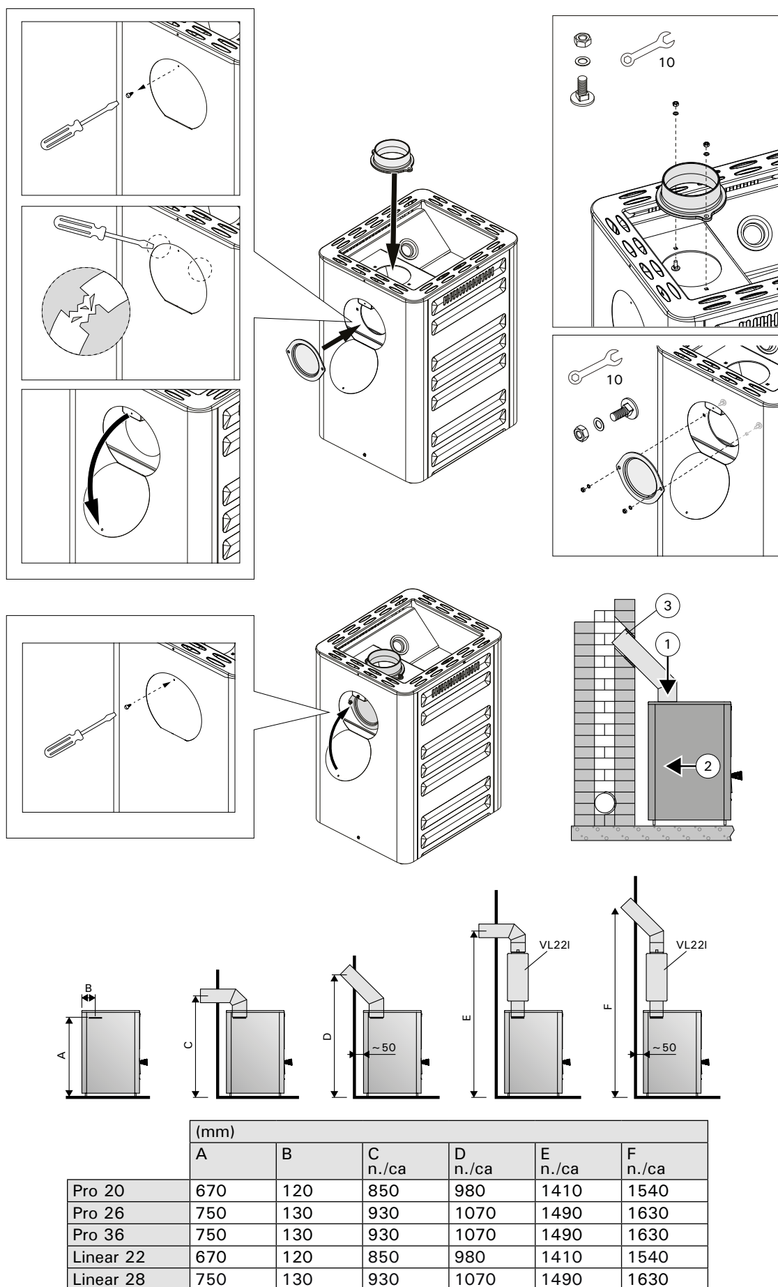
Obrázek 10. Připojení kamen ke zděří ve zdi z horního otvoru (všechny rozměry jsou uvedené v milimetrech) Figuur 10. De kachel aansluiten op een gemetseld rookkanaal via de aansluitopening boven (alle afmetingen in millimeters)
