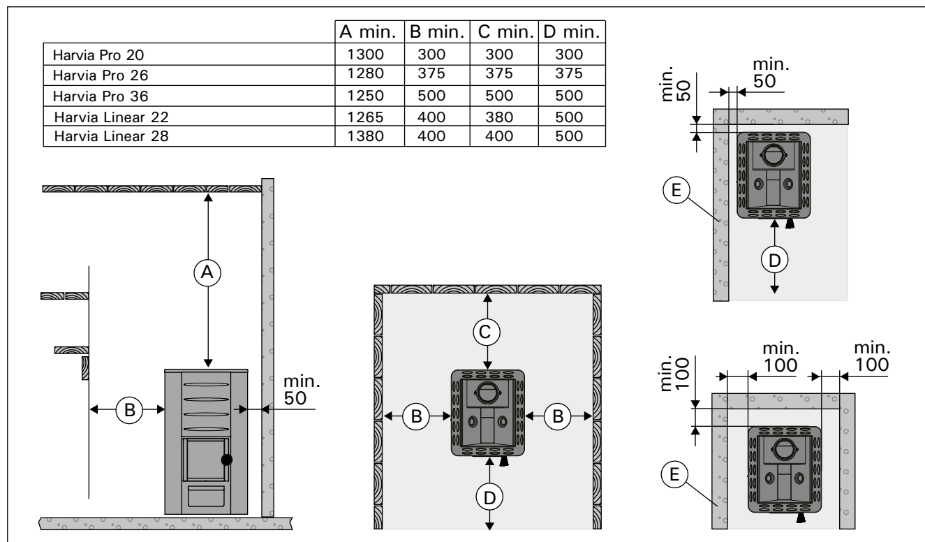
Figure 7. Distances de sécurité (toutes les dimensions sont fournies en millimètres)
