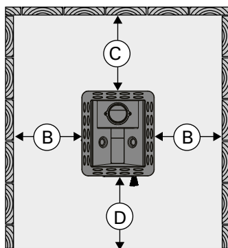
Obrázek 7. Bezpečné vzdálenosti pro topné těleso (všechny rozměry jsou uvedené v milimetrech) Figuur 7. Veiligheidsafstanden (alle afmetingen in millimeters)
