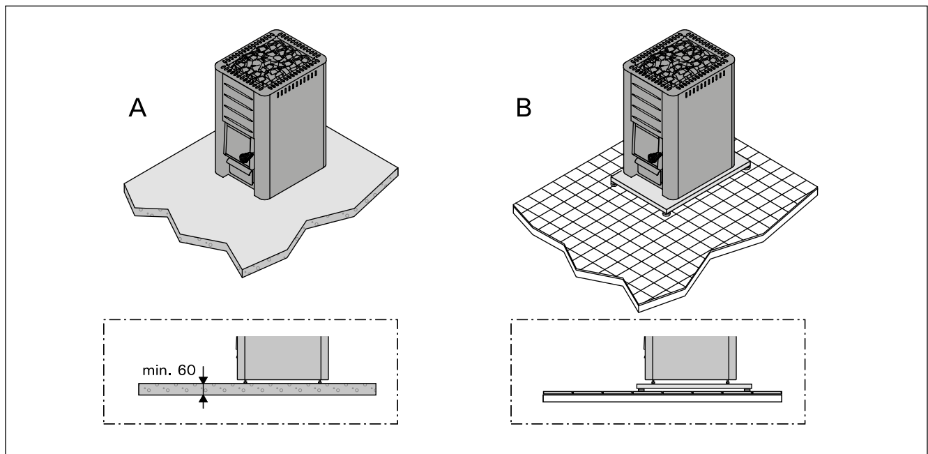
Kuva 6. Lattian suojaaminen (mitat millimetreinä)
