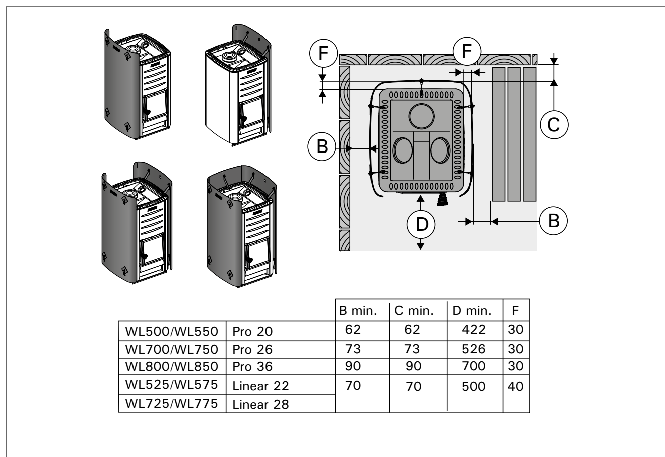
Figure 8. Distances de sécurité avec les gaines de protection (toutes les dimensions sont fournies en millimètres)
