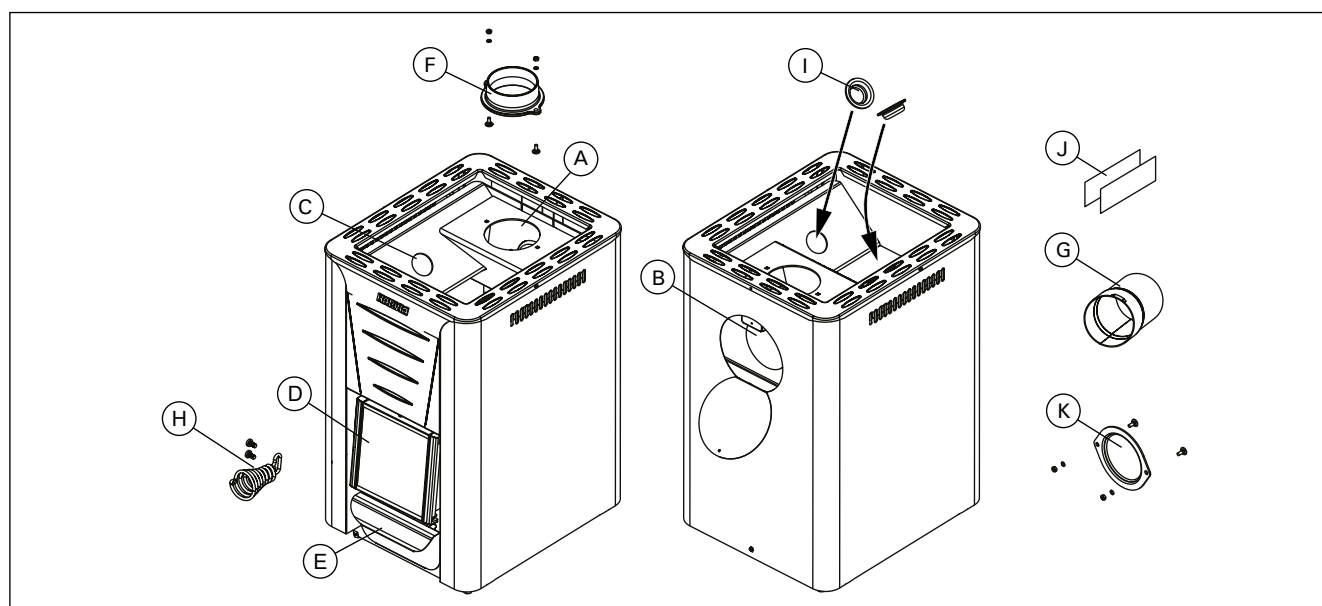
Figure 1. Composants du poêle. Toute modification du poêle sans autorisation est interdite.
